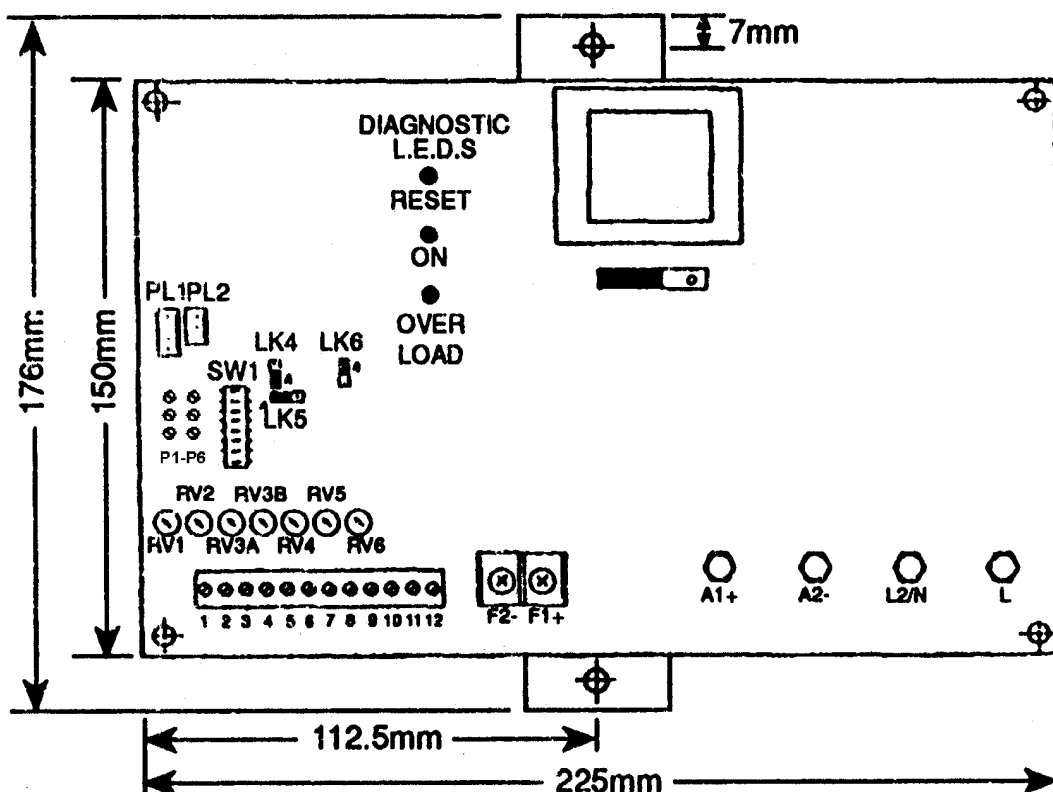
Рис. 1 Общий вид привода SHEETAN SM
