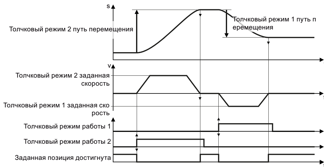
Изображены Инкрементальная толчковая подача е 8-35
