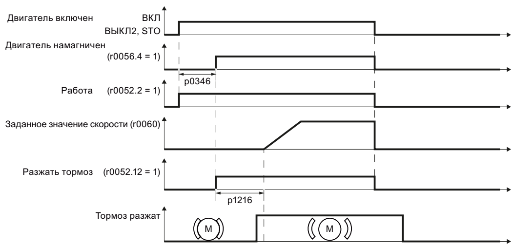
Изображены Управление стояночным тормозом двигателя после команды ВЫКЛ2 или выборе 8-44 STO
