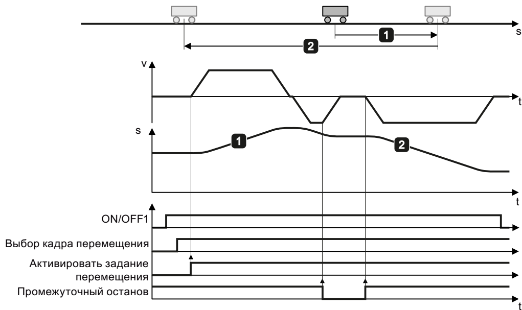
Изображены позиционирование оси через кадры перемещения 8-37
