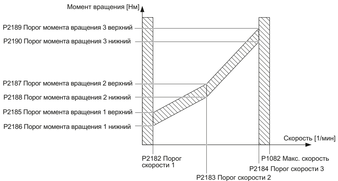
Изображены Параметры для контроля момента нагрузки е 8-45
