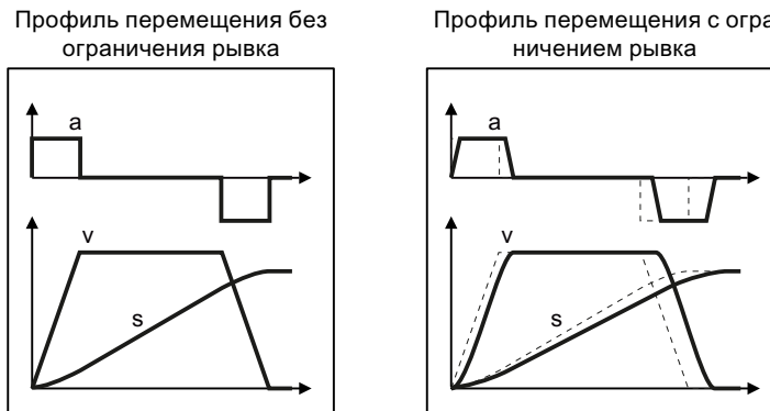
Изображены Пример: Действие ограничения рывка е 8-23
