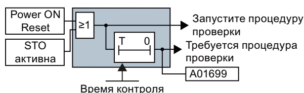
Изображены Запуск и контроль процедуры проверки е 8-51
