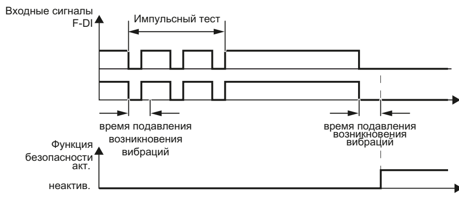
Изображени Фильтр для подавления короткого переключения сигнала е 8-50
