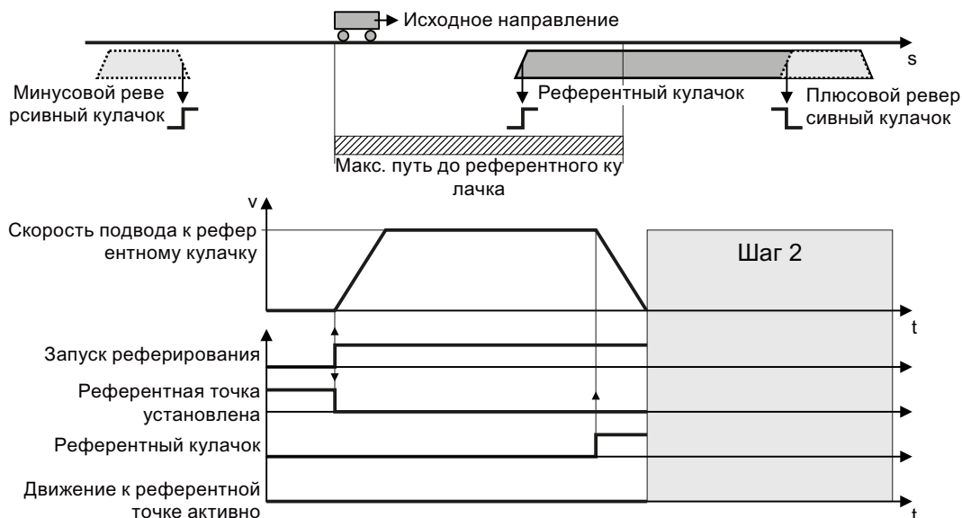
Изображение Шаг 1: Движение к референтному кулачку е 8-27
