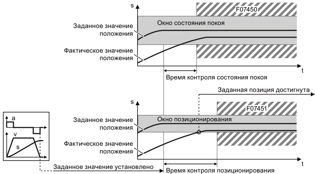
Изображены Контроль покоя и позиционирования е 8-24
