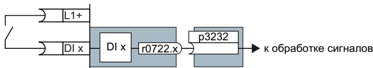
Изображени Контроль на предмет потери нагрузки посредством цифрового входа е 8-46
