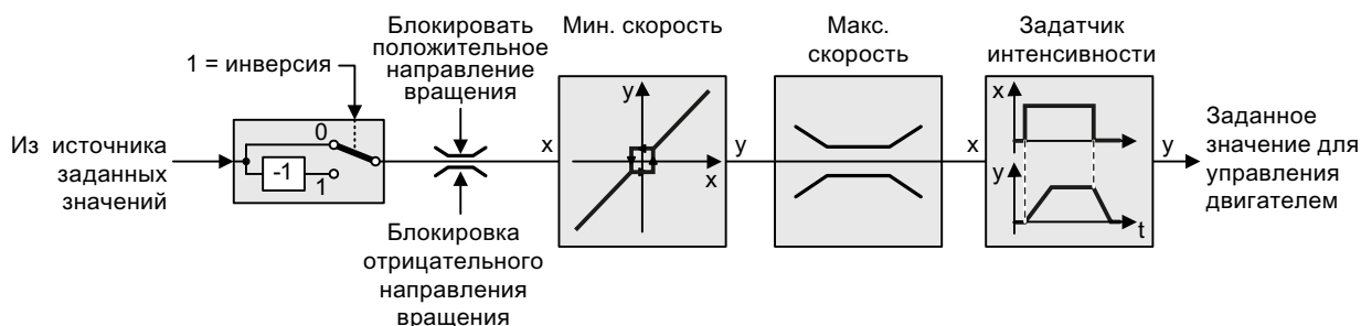
Изображены Подготовка заданного значения в преобразователе е 8-13
