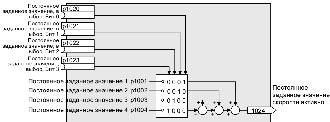
Изображени Упрощенная функциональная схема при прямом выборе постоянных заданных значений е 8-12
