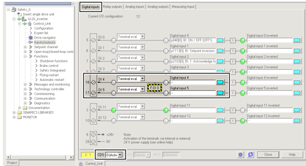
Изображены Удаление предустановки цифровых входов DI 4 и DI 5 е 8-53
