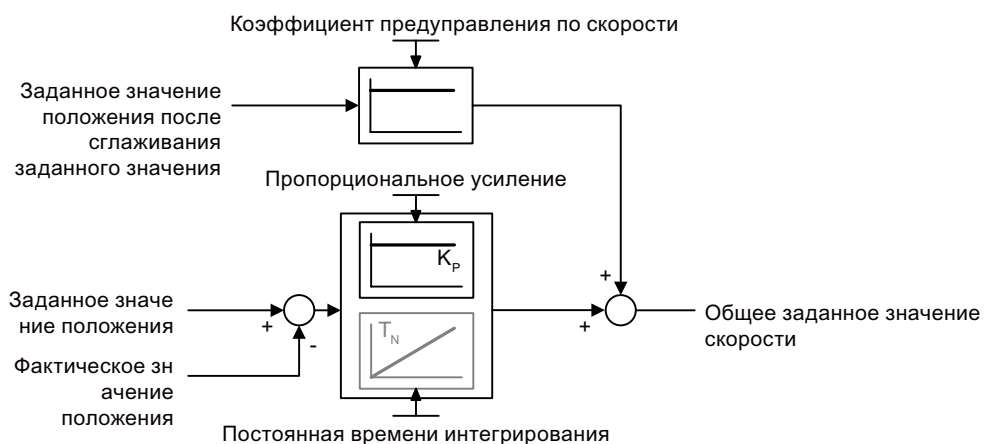
Изображени Регулятор положения с предупредлением е 8-22
