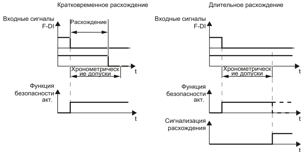
Изображены Допуск для расхождения e 8-48
