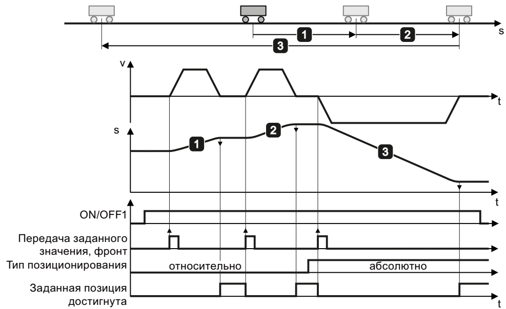
Изображены Позиционирование оси с прямой установкой заданного значения (MDI) е 8-39
