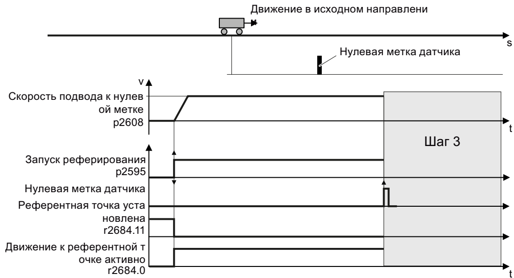
Изображены Движение к нулевой метке при отсутствии референтного кулачка е 8-29
