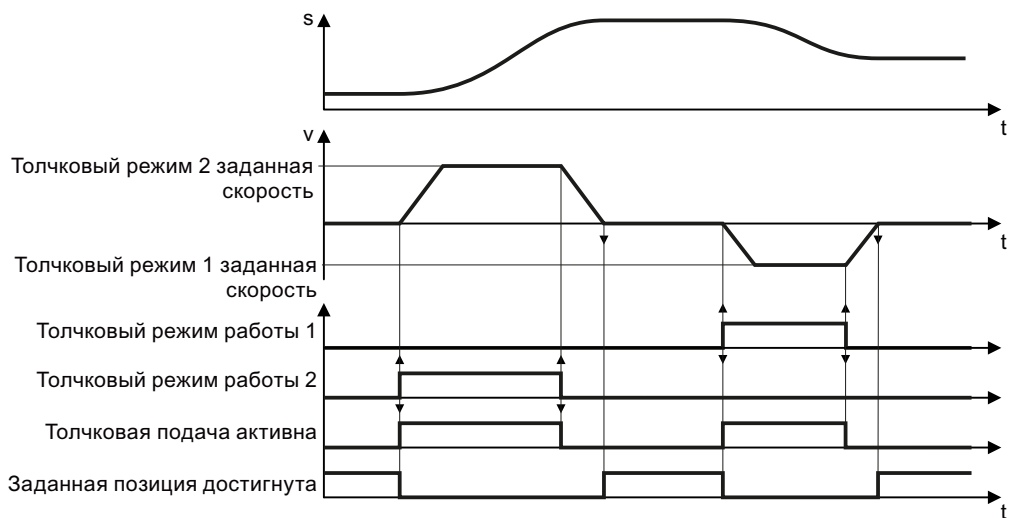
Изображени Скорость толчковой подачи е 8-34
