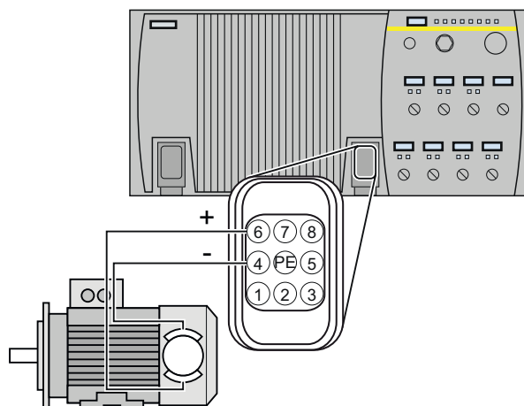
Изображены Упрощенная схема соединения СТД е 8-42
