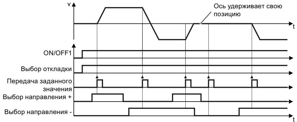
Изображены Отладка оси с прямой установкой заданного значения (MDI) е 8-40
