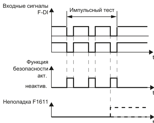
Изображени Реакция преобразователя на импульсный тест е 8-49
