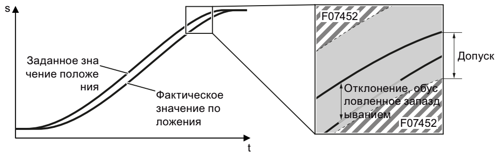
Изображены Контроль отклонения, обусловленного запаздыванием 8-25
