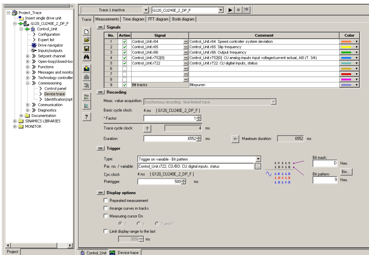
Изображены Диалоговое окно трассировки е А-12
