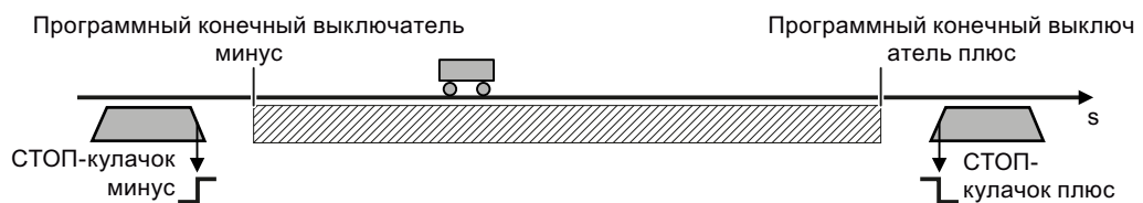
Изображены Ограничение области позиционирования линейной оси е 8-21
