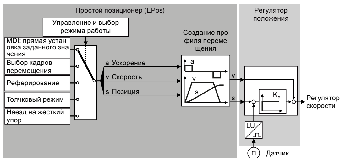
Изображены Простой позиционер и управление по положению е 8-18
