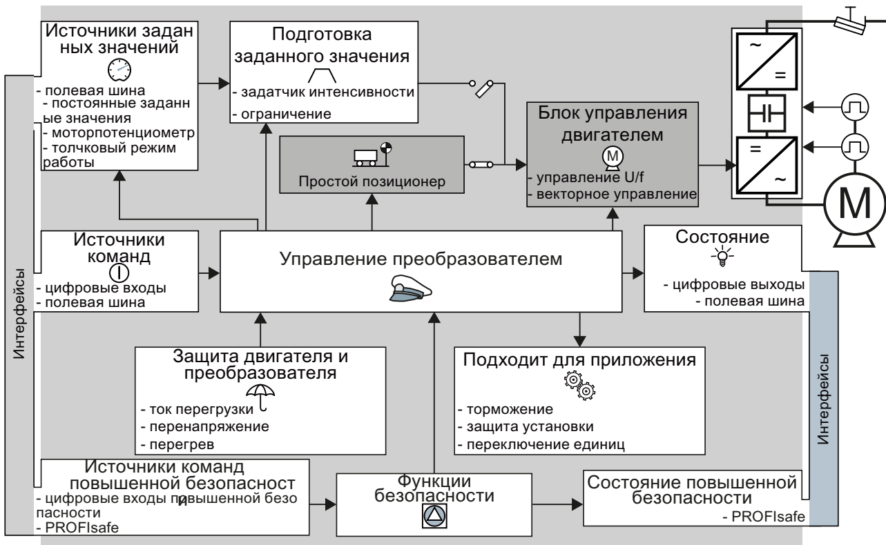
Изображение 8-1 Обзор функций в преобразователе
