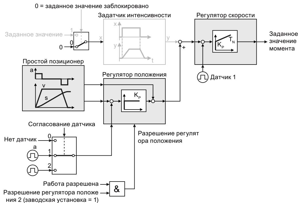
Изображены установка заданного значения для регулятора скорости в заводской установке преобразователя
