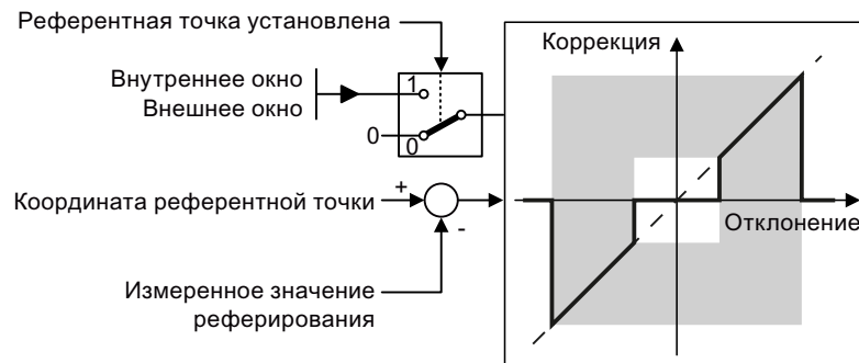
Изображены Внешнее и внутреннее окно при реферировании на лете е 8-32
