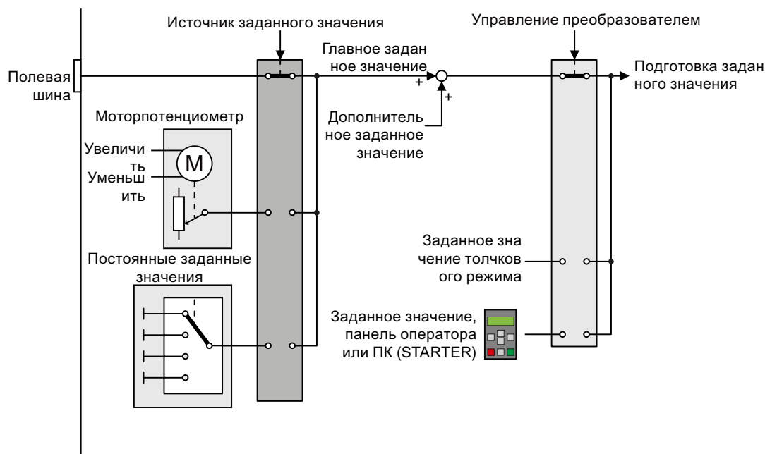
Изображены Источники заданных значений преобразователя е 8-7
