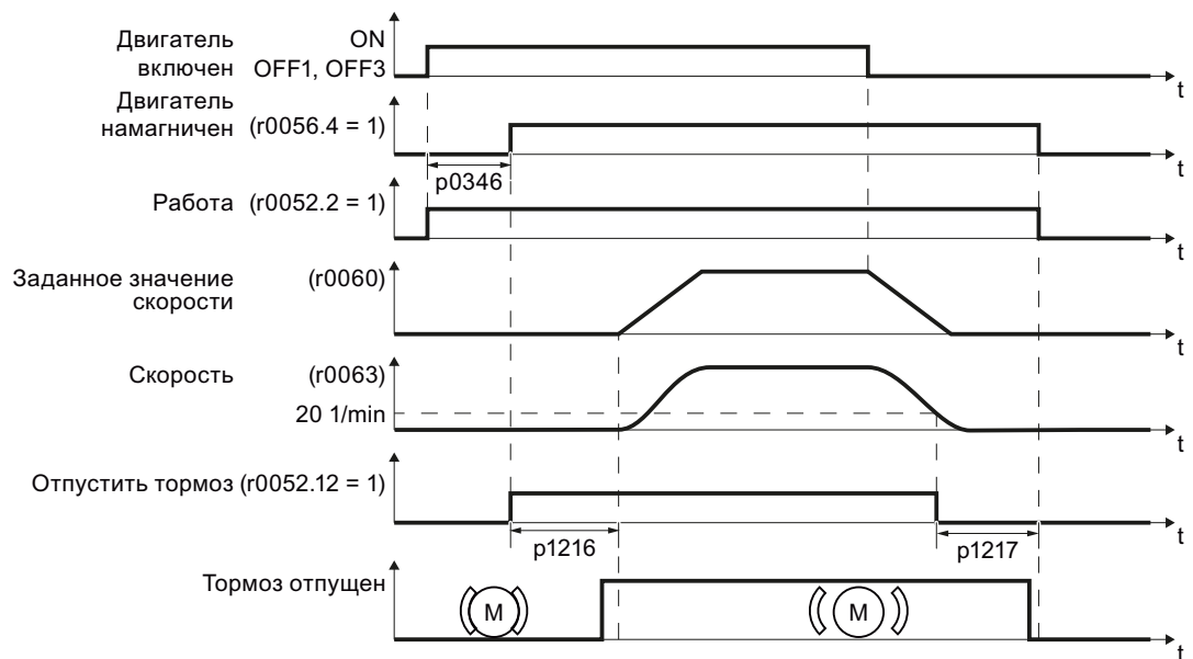
Изображены Управление стояночным тормозом двигателя при включении и выключении е 8-43 двигателя
