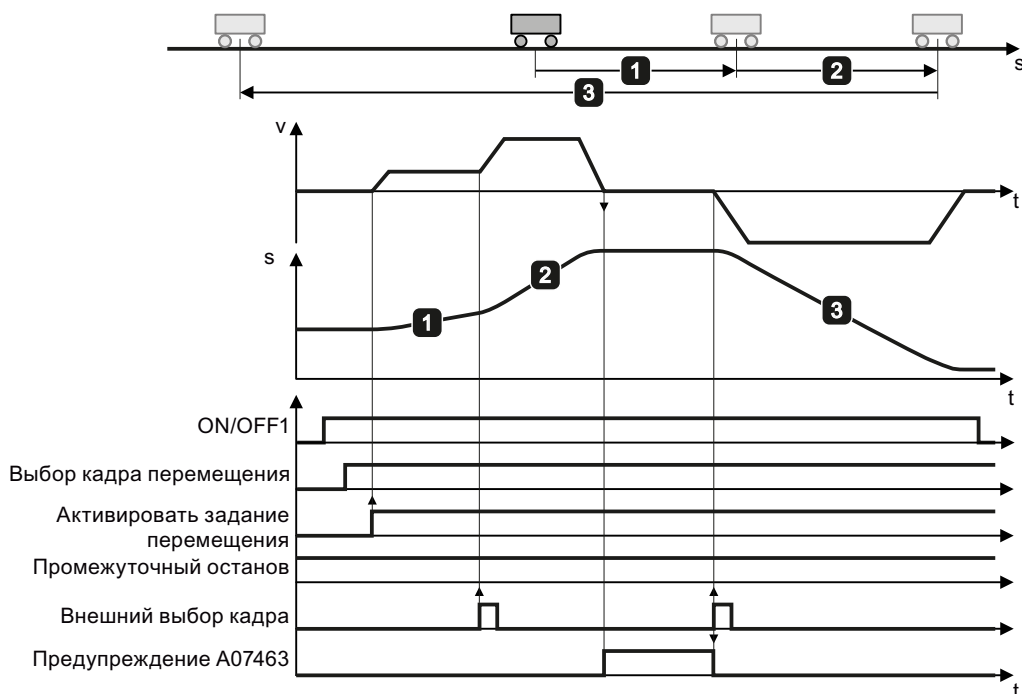
Изображены Позиционирование оси через кадры перемещения е 8-38
