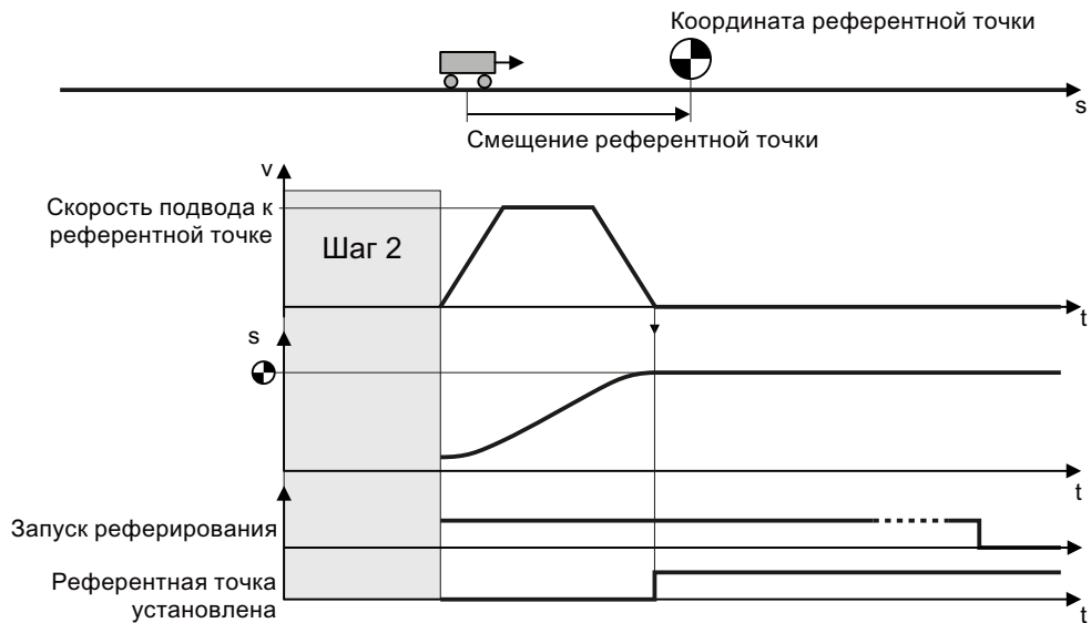
Изображены Шаг 3: Движение к референтной точке е 8-30
