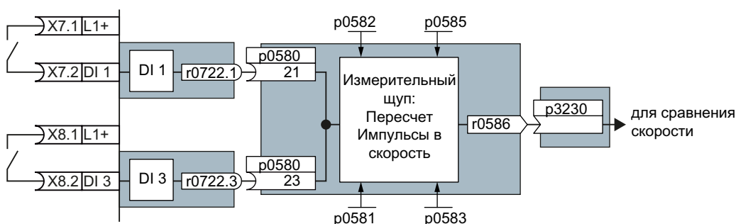
Изображени Контроль на предмет отклонения скорости вращения с помощью цифрового входа е 8-47 DI 1 или DI 3
