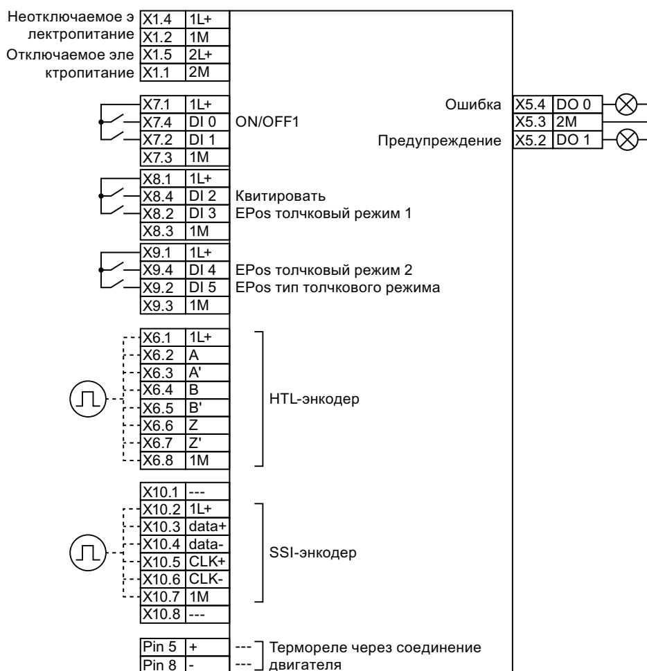
Изображены Подключение согласно заводской установке привода е 5-2
