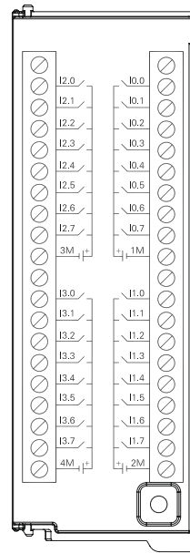
SM3DI32
