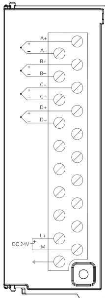
AIT-04
