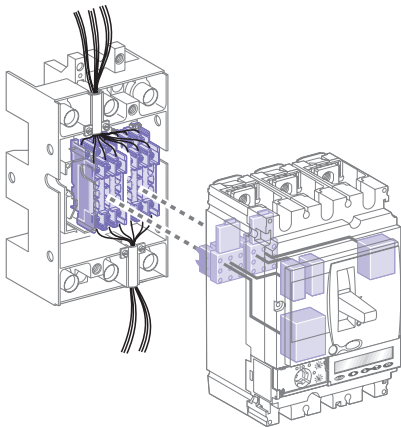
Втычной/выдвижной аппарат SystemePact CCB
