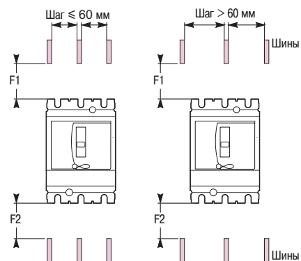
Сборные шины под напряжением
