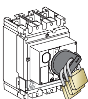
Блокировка поворотной рукоятки навесным замком
