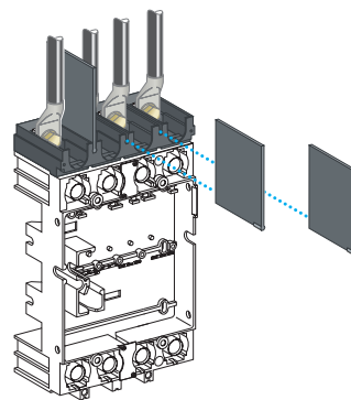
Переходник для цоколя 4-полюсного аппарата 400/630 А. Присоединение расширителей полюсов с разделителями полюсов
