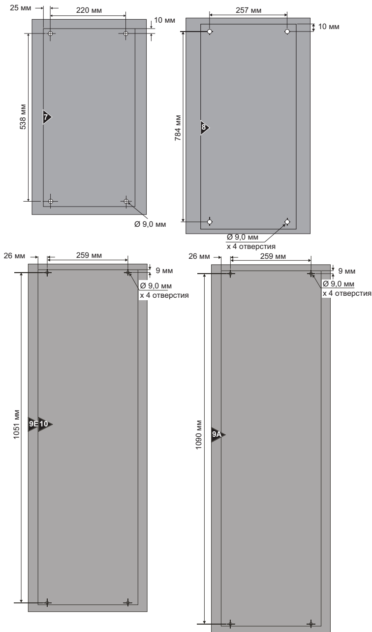
Рис. 3-2 Размеры при монтаже на поверхности (габариты 7 до 10)
