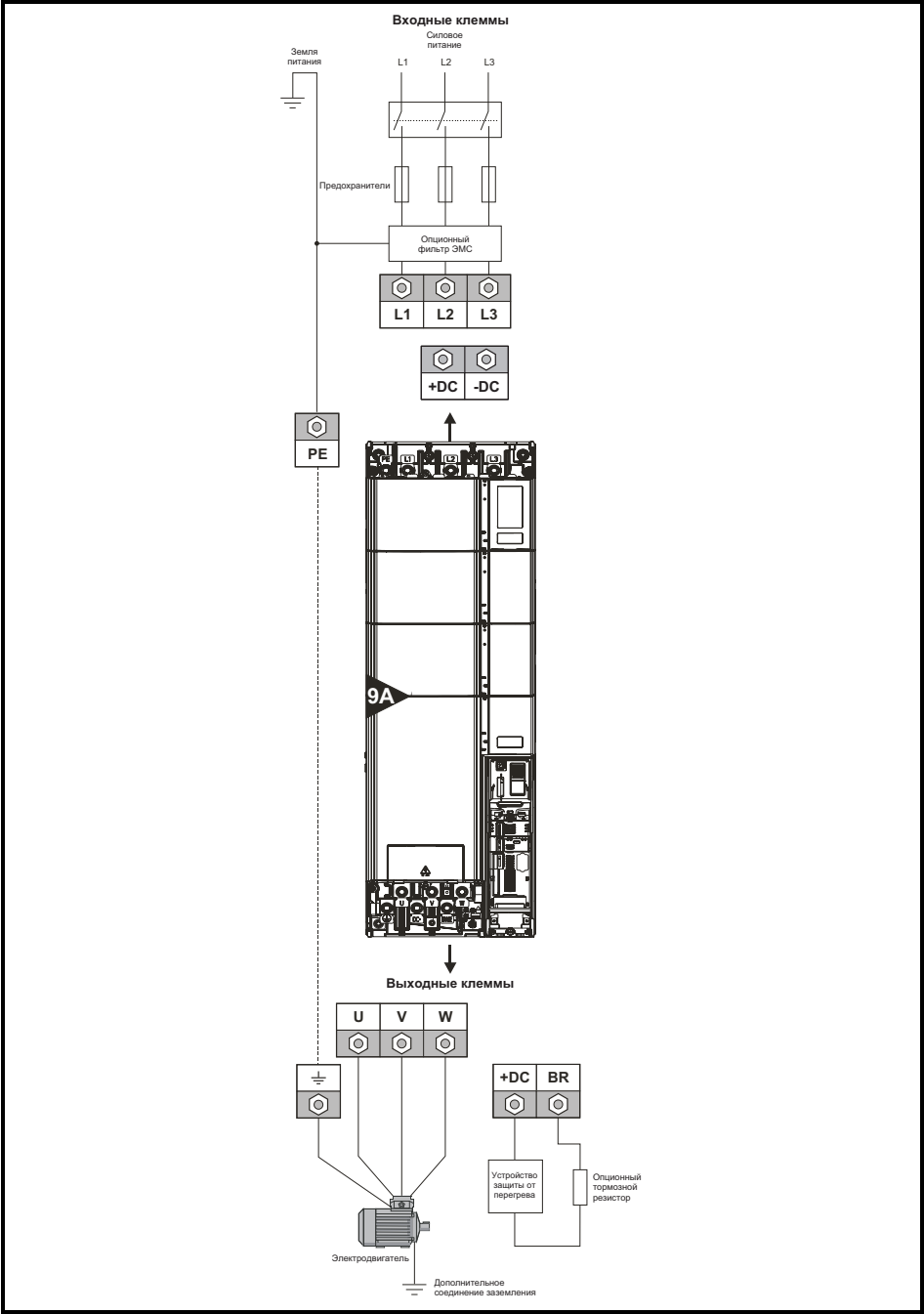
Рис. 4-2 Подключение питания и заземления к габариту 9A
