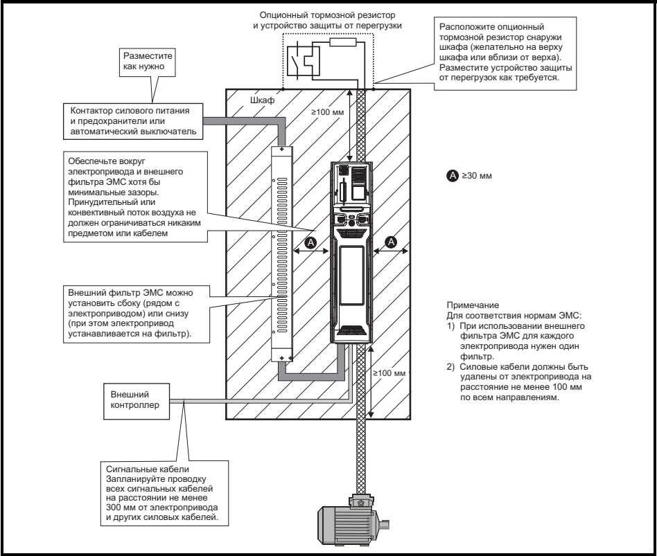
Рис. 3-4 Компоновка шкафа
