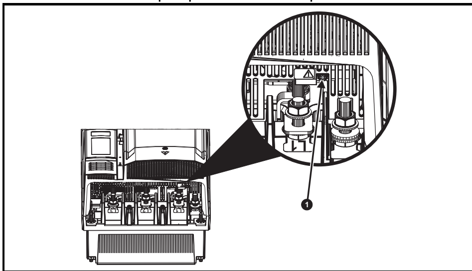
Рис. 3-6 Снятие линии на варисторы заземления на габарите 9Е и 10
